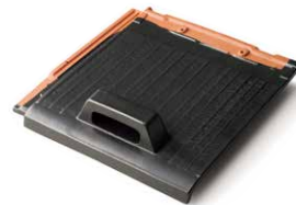
雪止瓦 対応色:瓦全色
